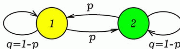
Рис. 5.6. Диаграмма Мура автомата с двумя состояниями
