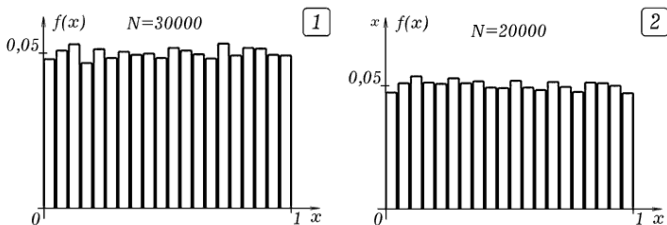
Рис. 5.2. Практически равномерные распределения случайных чисел
