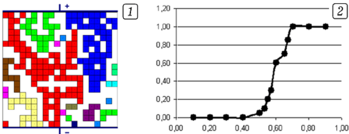
Рис. 5.5. Изучение перколяции методом статистического моделирования
