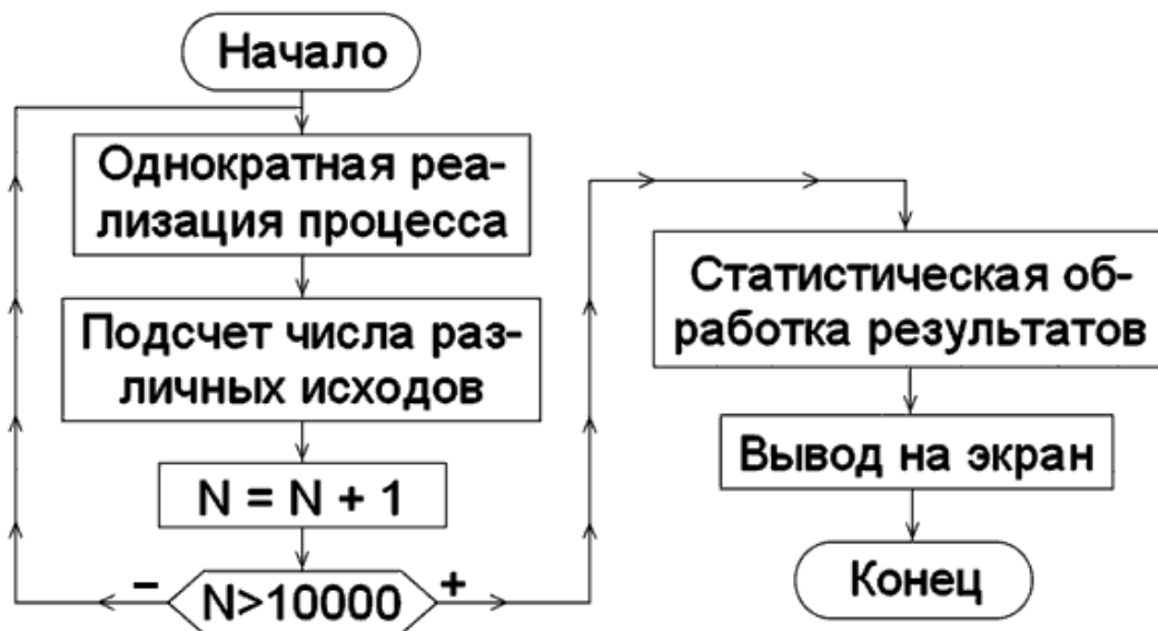
Рис. 5.1. Сущность метода статистических испытаний
