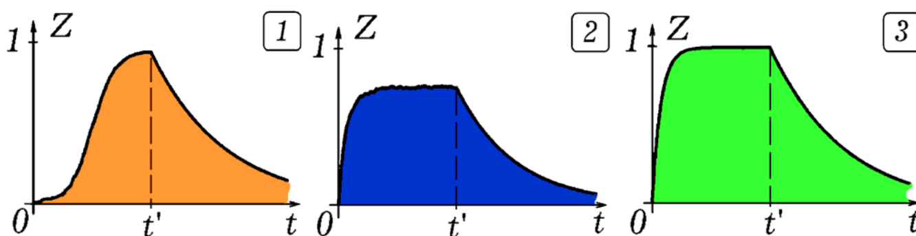
Рис. 5.7. Зависимости уровня знаний "ученика" от времени
