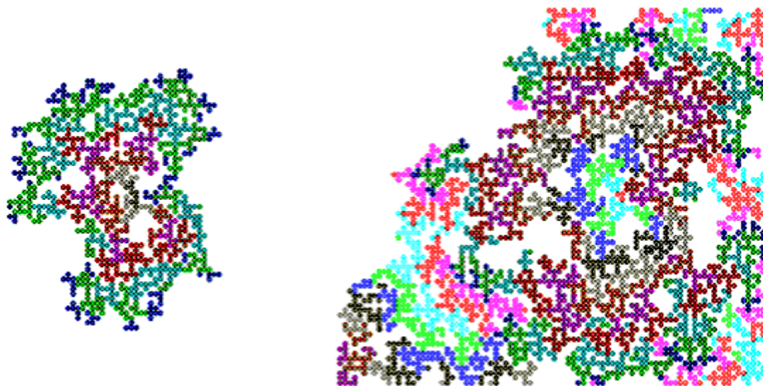
Рис. 5.10. Стохастический фрактал
