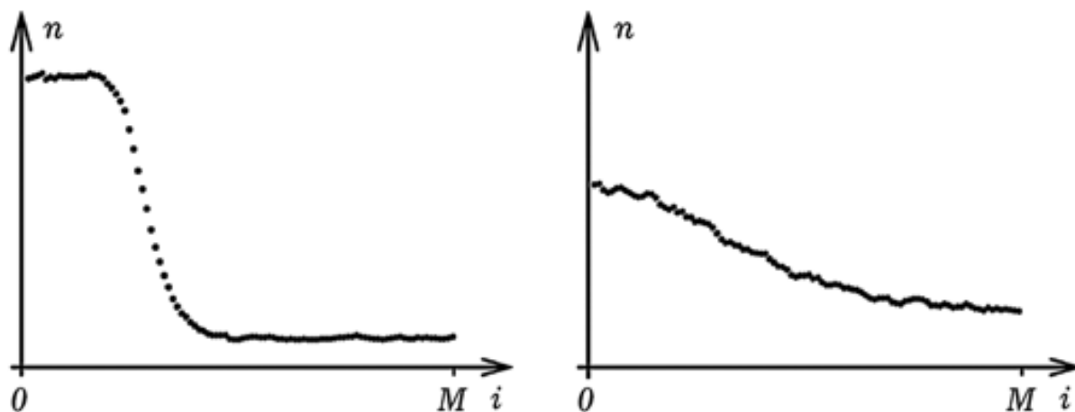
Рис. 5.8. Моделирование диффузии с помощью вероятностных КА
