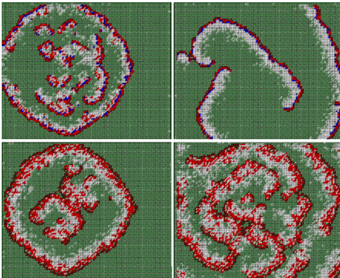
Рис. 5.9. Рост колонии бактерий: вероятностный КА
