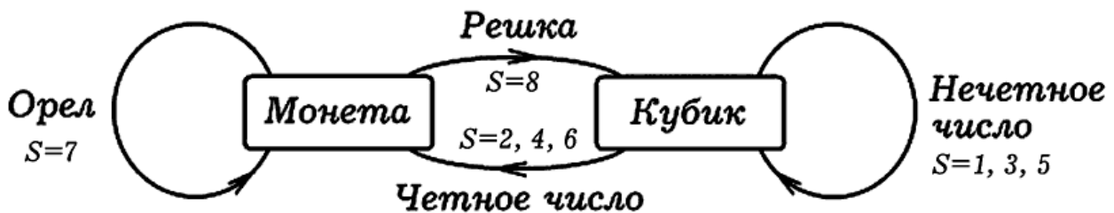
Рис. 5.4. Граф, описывающий смену состояний системы
