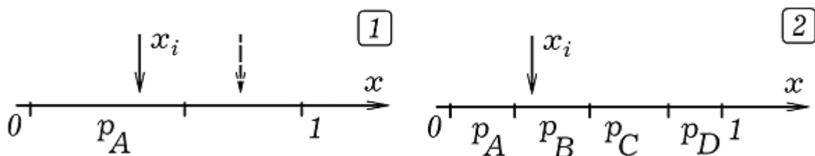
Рис. 5.3. Метод определения исходов по жребию
